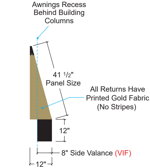
SE Side Elevation Scale: 3/8" = 1'
