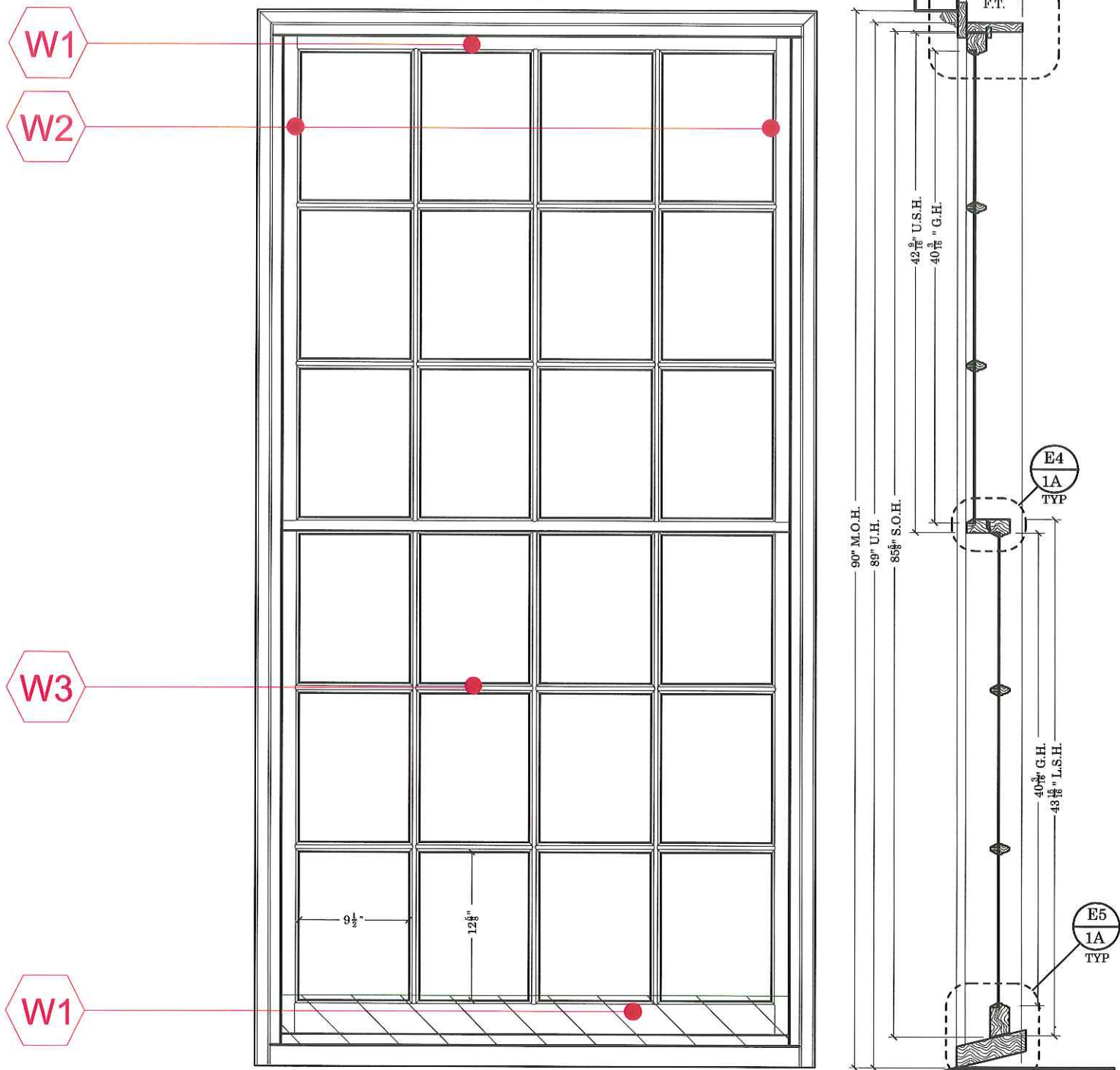
ELEVATION
