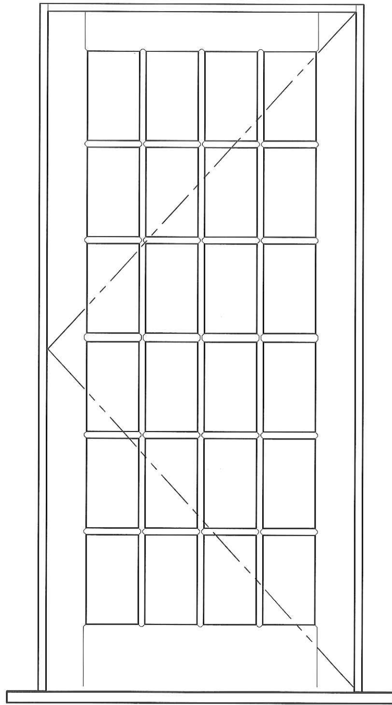
ELEVATION
